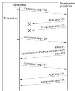
Диаграмма последовательности операций при потере возвратного сообщения)
